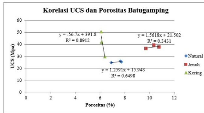
Gambar 10 Korelasi UCS Dan Porositas Batugamping
