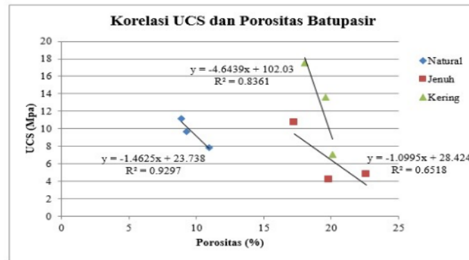
Gambar 13 Korelasi UCS Dan Porositas Batupasir
