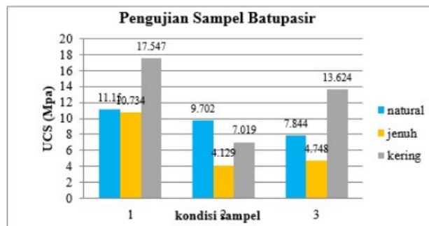
Gambar 8 Perbandingan Hasil Uji Kuat Tekan Pada Batupasir.
