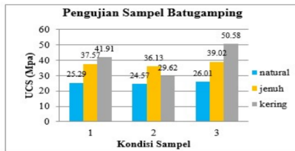
Gambar 7 Perbandingan Hasil Uji Kuat Tekan Pada Batugamping
