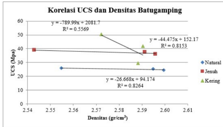
Gambar 11 Korelasi UCS Dan Densitas Batugamping
