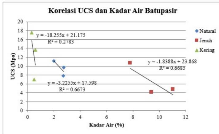
Gambar 12 Korelasi UCS Dan Kadar Air Batupasir
