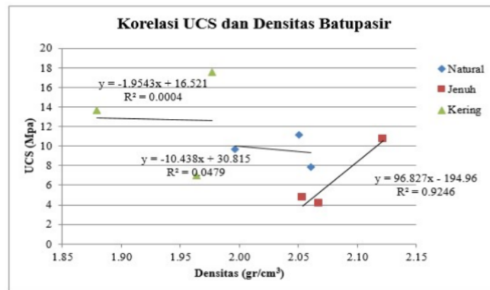
Gambar 14 Korelasi UCS Dan Densitas Batupasir
