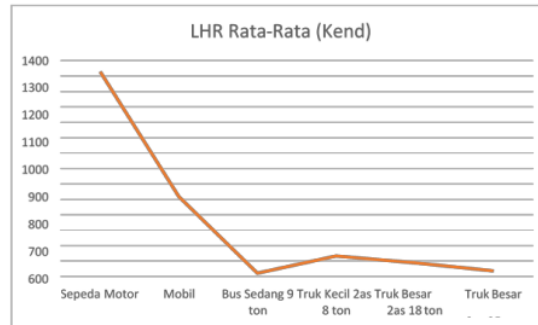
Gambar 5 Grafik LHR
