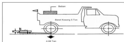
Gambar 1. Truk yang dipergunakan untuk servey lendutan
