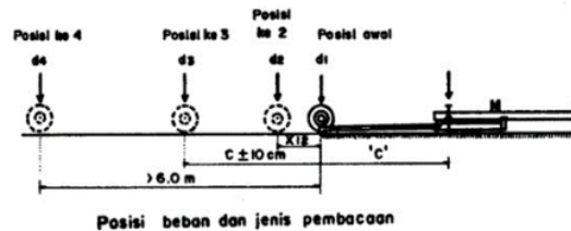
Gambar 4. Posisi dan jenis pembacaan
