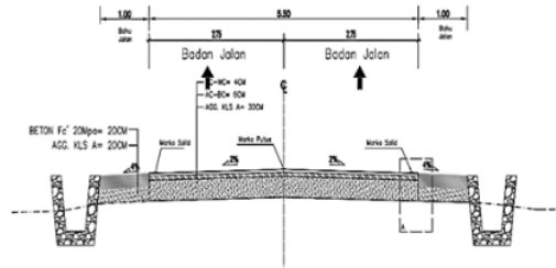
Gambar 6 Sketsa rencana potongan melintang jalan baru
