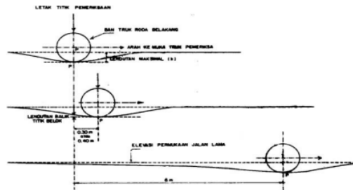
Gambar 3 Hubungan antara lendutan dengan pembebanan
