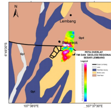
7 Gambar 4. Peta Overlay Geologi dengan Anomali Magnet Total.
