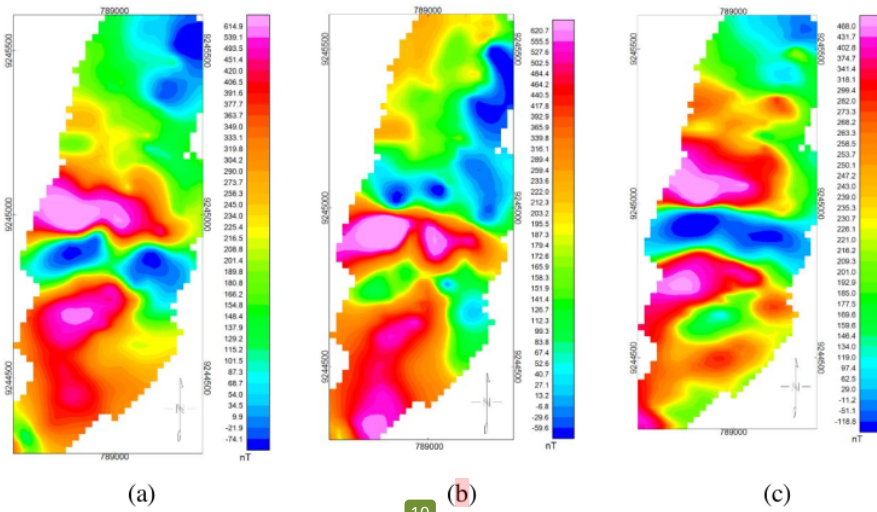
10 Gambar 3. Anomali magnet total (a), Reduksi ke Kutub (b), Reduksi ke Ekuator (c)
