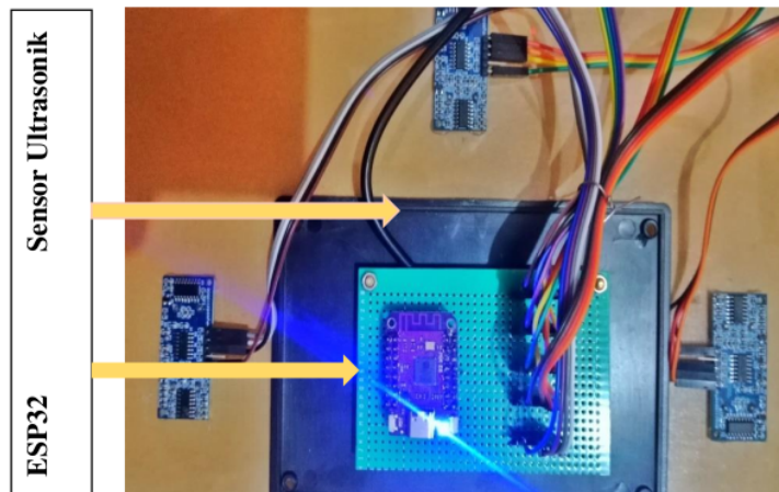
Gambar 13 Pengujian ESP32
