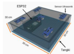
Gambar 10. Desain Alat Sumber : Dokumen Pribadi
