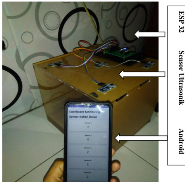
Gambar 14. Pengujian sensor ultrasonik
