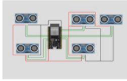
Gambar 11. Skema Wiring Perancangan Alat
