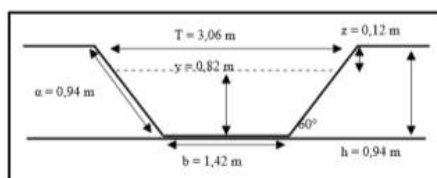
Gambar 4. Rancangan Dimensi Saluran Terbuka
