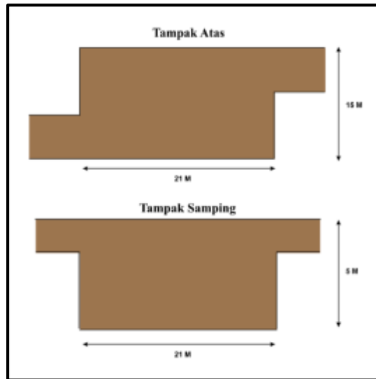
Gambar 5. Rancangan Dimensi Kolam Pengendapan
