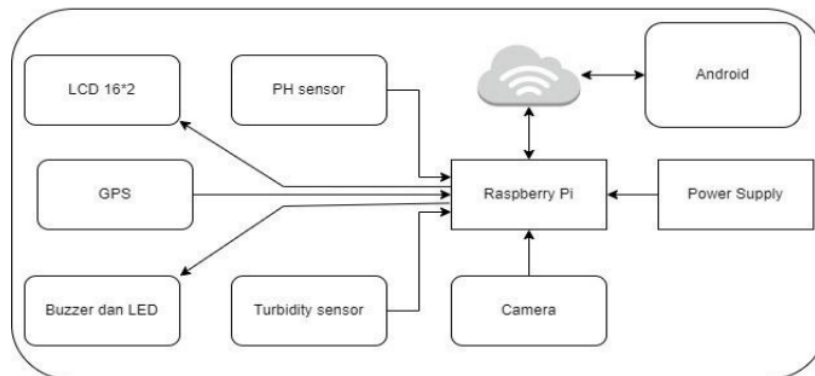
Gambar 1. Diagram blok sistem yang dirancang
