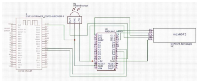
Gambar 1. Wiring Diagram Perancangan Alat
