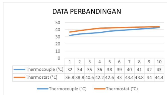
Gambar 6. Grafik Perbandingan Pengukuran Suhu Ketika Alat ON
