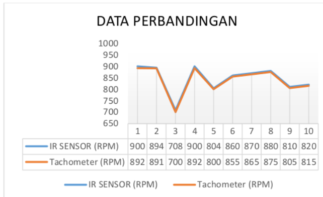
Gambar 5. Grafik Perbandingan Pengukuran RPM
