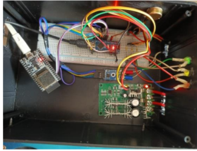
Gambar 9. Alat Tampak Dalam
