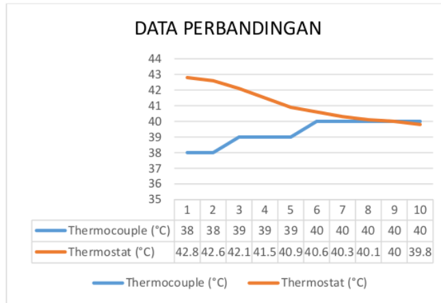
Gambar 7. Grafik Perbandingan Pengukuran Suhu Ketika Alat OFF
