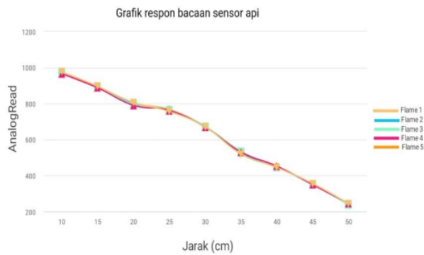
Gambar 4. Grafik Pembacaan Setiap Flame Sensor
