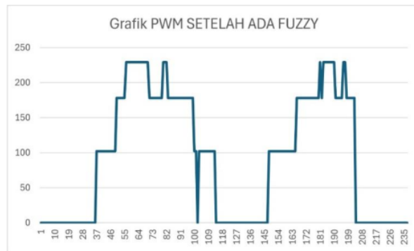
Gambar 11. Grafik Pengujian PWM Setelah Ada Fuzzy
