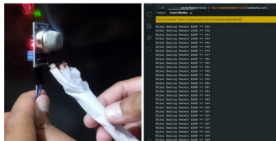
24 Gambar 4. Pengujian Sensor Asap MQ-2
