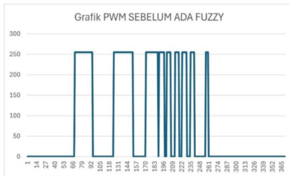
Gambar 10. Grafik Pengujian PWM Sebelum Ada Fuzzy
