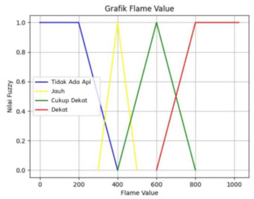
Gambar 9. Membership Fuction Pada Api
