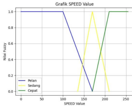
Gambar 9. Membership Fuction Pada PWM Driver Mosfet
