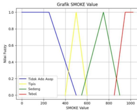
Gambar 8. Membership Fuction Pada Asap
