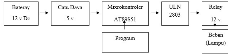
Gambar 1 Diagram blok Sistem Kerja Rangkaian Smart Relay
