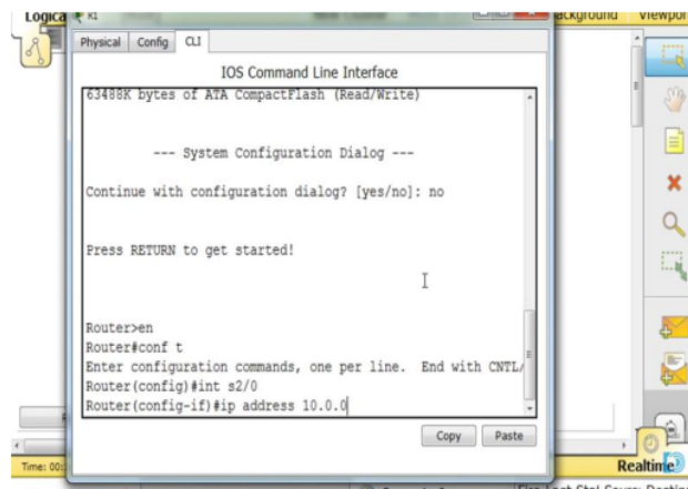
Gambar 5. Program Router Pada Command Line Interface (CLI)
