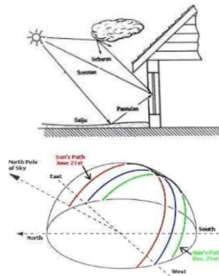
Gambar 2- 2. Lintasan tahunan matahari sumber: (Rifan et al., 2012)
