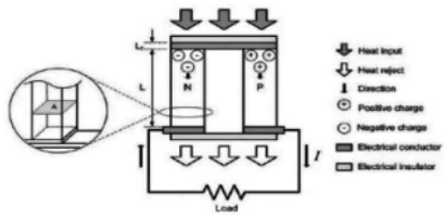
Gambar 2 – 4. Skema kinerja generator termoelektrik.
