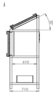
Gambar 2-5. Desain alat simulasi penelitian
