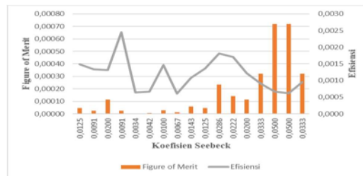
Gambar 4-5 Pengaruh koefisien Seebeck terhadap figure of merit dan efisiensi pada rangkaian paralel
