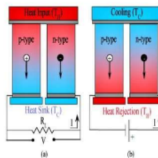
2 Gambar 2 - 3. Pengaturan modul termoelektrik untuk (a) pembangkit listrik oleh efek Seebeck dan (b) pendinginan oleh efek Peltier.
