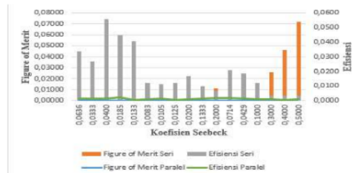
Gambar 4-7 Pengukuran terhadap figure of merit, koefisien Seebck, dan efisiensi pada rangkaian seri dan paralel
