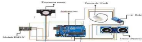
Gambar 14 Perancangan Alat Sumber: Dokumen Pribadi
