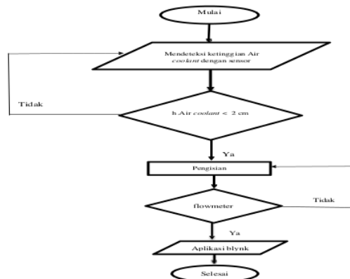
Gambar 13 Diagram Alir Perancangan Sistem Sumber: Dokumen Pribadi
