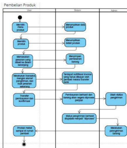
Gambar 3. Activity Diagram Pembelian Produk
