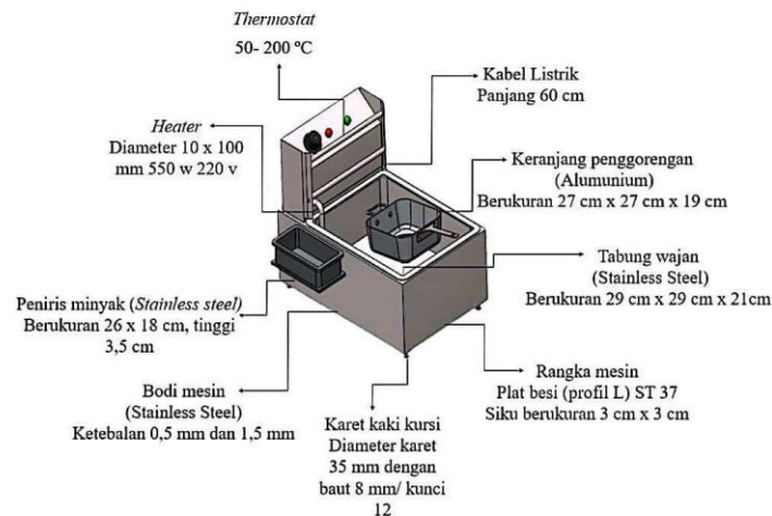
Gambar 5 Skema Desain Rancang Bangun Mesin Penggorengan Chicken Dengan Metode Deep Fryer
