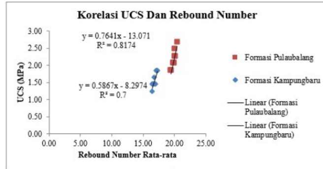
Gambar 10 Grafik korelasi UCS dengan Rebound Number
