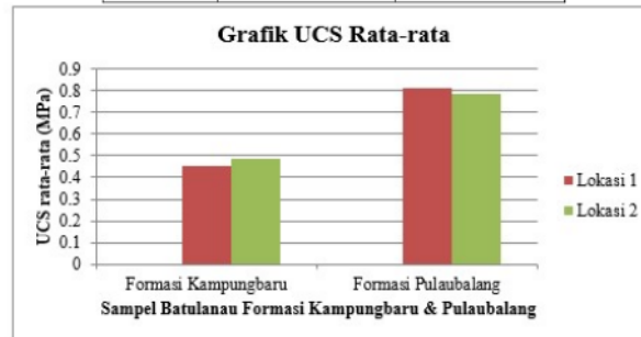
Gambar 6 Grafik nilai UCS
