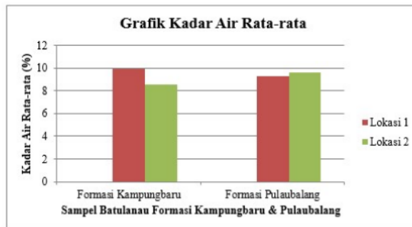
Gambar 1 Grafik kadar air rata-rata batulanau Formasi Kampungbaru dan Pulaubalang
