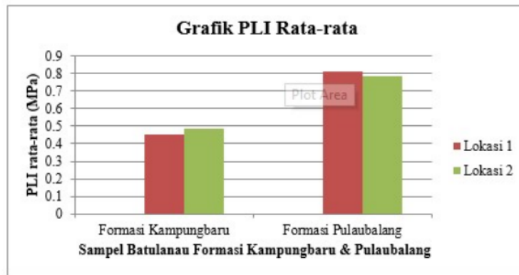
Gambar 5 Grafik nilai PLI
