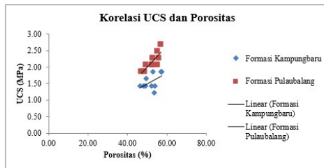
Gambar 8 Grafik korelasi UCS dengan porositas
