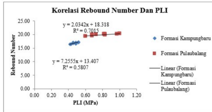
Gambar 12 Grafik korelasi rebound number dan PLI
