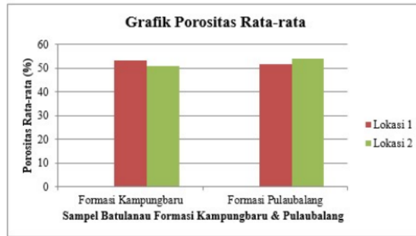
Gambar 2 Grafik porositas rata-rata batulanau Formasi Kampungbaru dan Pulaubalang
