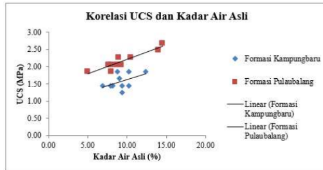
Gambar 9 Grafik korelasi UCS dengan kadar air asli
