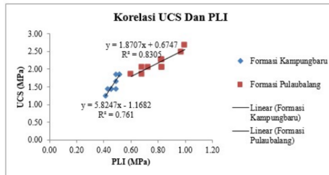
Gambar 11 Grafik korelasi UCS dan PLI
