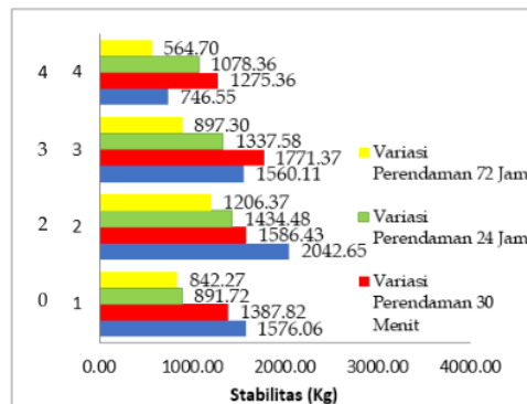
Gambar 6. Hubungan antara Presentase Limbah Ban Karet Bekas Dengan Stabilitas
