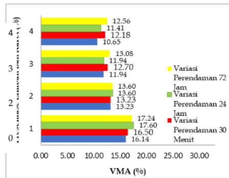
Gambar 4. Hubungan antara Presentase Limbah Ban Karet Bekas Dengan VMA
