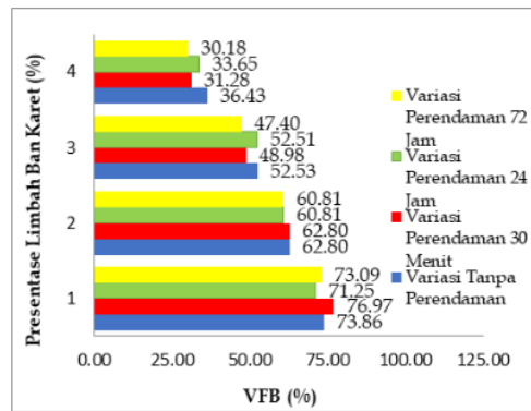
Gambar 5. Hubungan antara Presentase Limbah Ban Karet Bekas Dengan VFB
