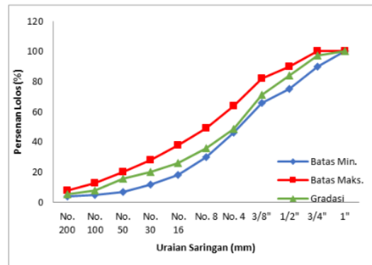
Gambar 1. Gradasi Campuran Aspal
