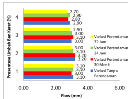
Gambar 7. Hubungan antara Presentase Limbah Ban Karet Bekas Dengan Flow
