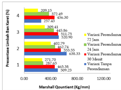
Gambar 8. Hubungan antara Presentase Limbah Ban Karet Bekas Dengan Marshall Qountient (Hasil Pengujian 2023)
