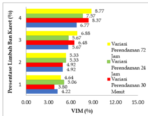
Gambar 3. Hubungan antara Presentase Limbah Ban Karet Bekas Dengan VIM
