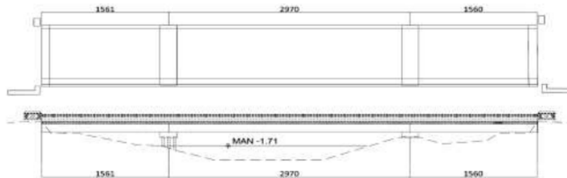
Gambar 2.2 Denah dan Tampak Samping Jembatan Maribaya A
