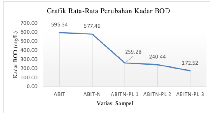
Gambar 3. Grafik Rata-Rata Perubahan Kadar BOD
