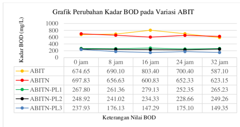
Gambar 2. Grafik Perubahan Kadar BOD pada Variasi ABIT
