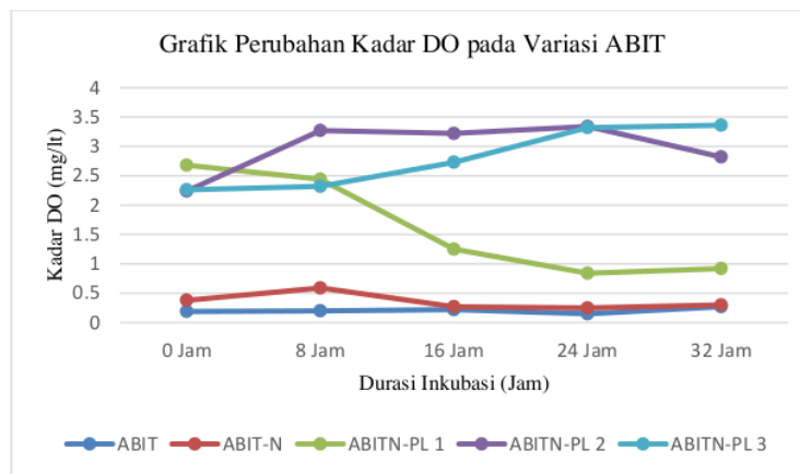
Gambar 1. Grafik Perubahan Kadar DO pada Variasi ABIT
