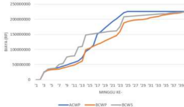
Gambar 4.3 Grafik Indikator Earned Value pada Minggu ke-40
