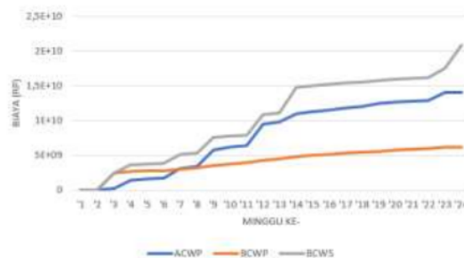
Gambar 4.2 Grafik Indikator Earned Value pada Minggu ke-24
