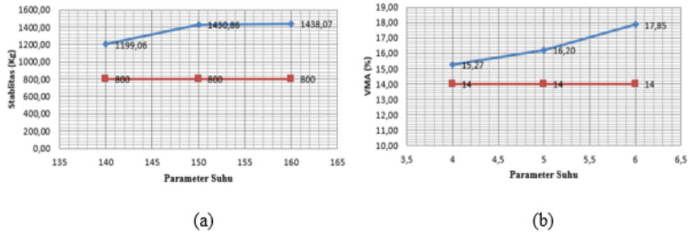
Gambar 2. (a). Hubungan suhu dan Stabilitas, (b) hubungan Suhu dan VMA
