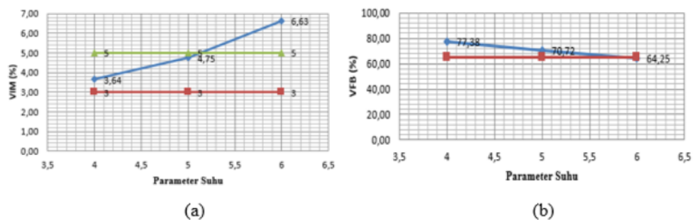
Gambar 3. (a) Hubungan Suhu dan VIM, (b) Hubungan suhu dan VFB
