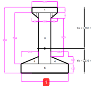
Gambar 23. Penampang balok sebelum komposit
