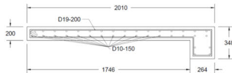
Gambar 20. Penulangan Plat Injak
