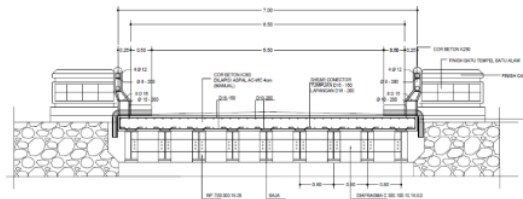
Gambar 3. Potongan melintang jembatan eksisting
