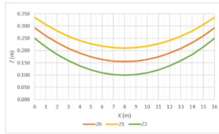
Gambar 28. Diagram posisi kabel be prategang
