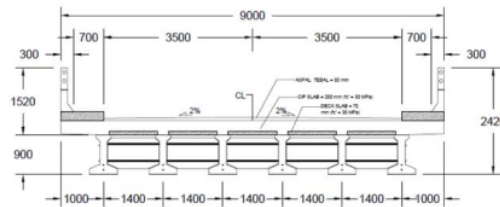
Gambar 7. Perencanaan ulang struktur atas jembatan
