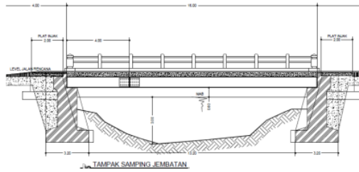
Gambar 2. Tampak samping jembatan eksisting
