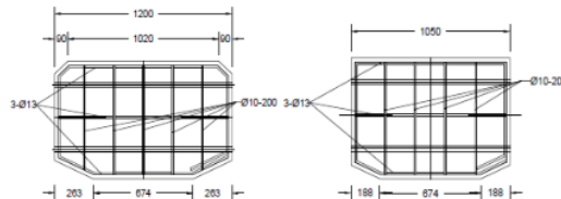
Gambar 21. Penulangan Diafragma
