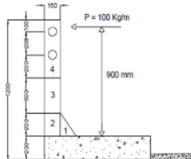
Gambar 8. Tiang dan Dinding Sandaran
