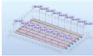
Gambar 12. Perletakan beban akibat berat sendiri (MS)
