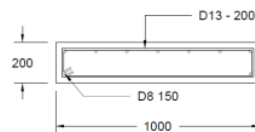
Gambar 11. Penulangan Trotoar
