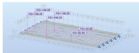
Gambar 16. Kondisi 1 beban truk
