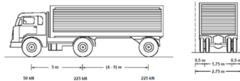
Gambar 15. Beban truk dan jarak antar gandar truk
