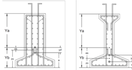
Gambar 27. Letak tendon pada tumpuan serta pada tengah bentang gelagar
