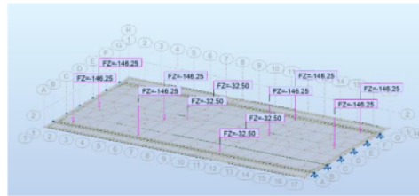
Gambar 18. Kondisi 3 beban truk
