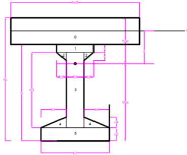
Gambar 24. Penampang balok setelah komposit
