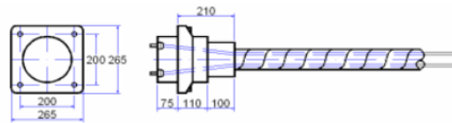
Gambar 29. Angkur hidup
