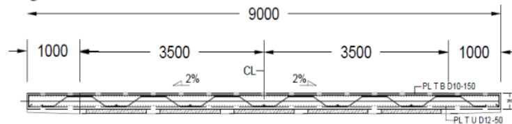
Gambar 19. Penulangan Plat Lantai
