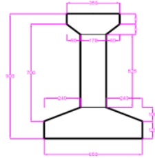
Gambar 22. Penampang Girder
