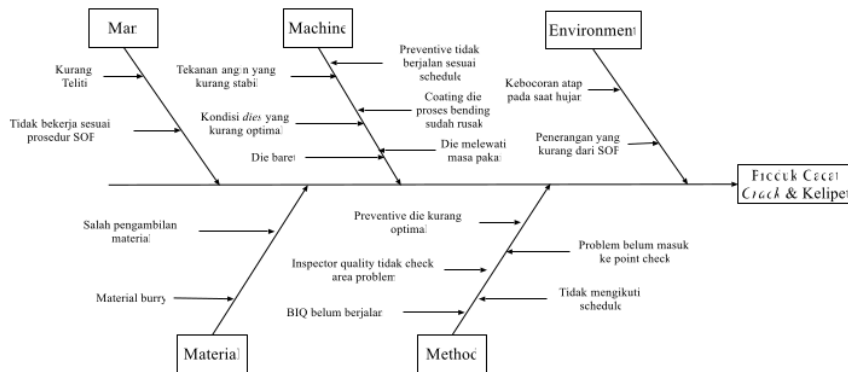
Gambar 5. Diagram Sebab Akibat Kecacatan Crack & Kelipet
