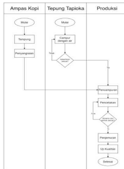
Gambar 9. Flowchart Produksi Briket
