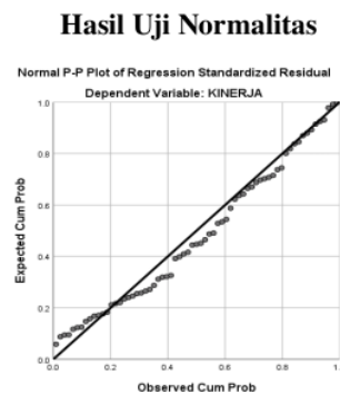
Gambar 4. 1 Uji Normalitas
