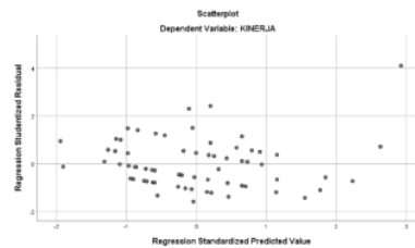
Gambar 4. 2 Uji Heteroskedastistas
