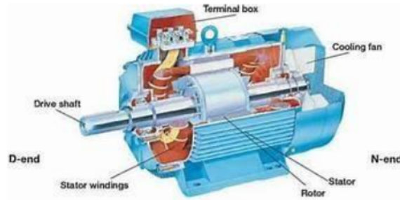
Gambar 2. Motor Induksi
