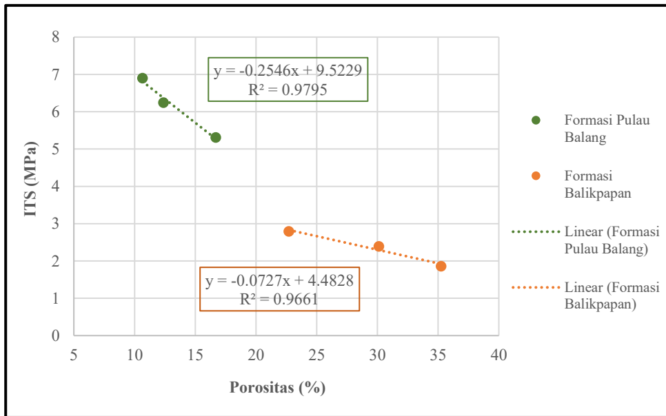
Gambar 6. Korelasi Porositas Terhadap Nilai ITS Kedua Formasi.
