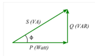
Gambar 3 Segitiga Daya
