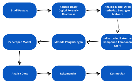
Gambar 2. Metodologi Penelitian.
