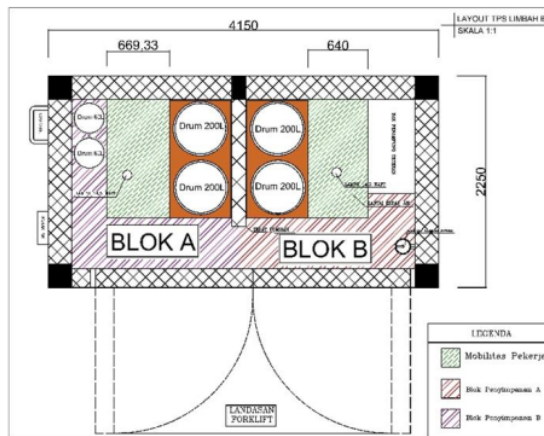
Gambar 1. Layout TPS Limbah B3 Baru
