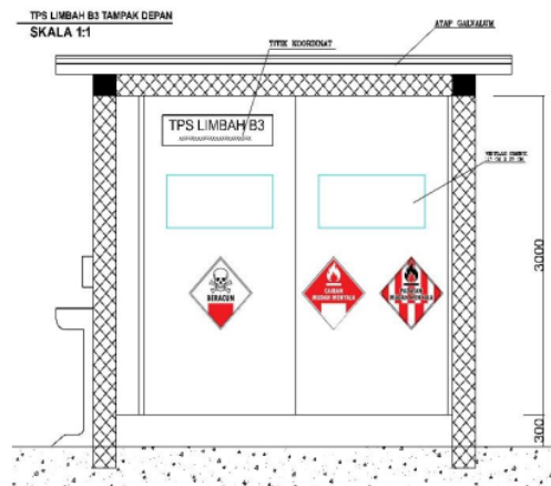
Gambar 2. Layout TPS Limbah B3 Baru
