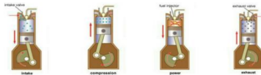
Gambar 2.1 Langkah Hisap – Langkah Buang Sumber: www.autoexpose.org
