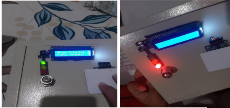
Gambar 4. 2 Pengujian Sensor RFID READER.
