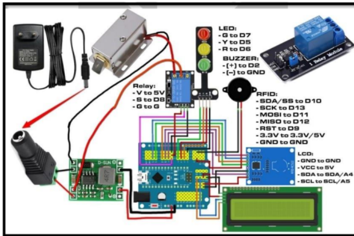
GAMBAR 3.3 Wiring perancangan alat
