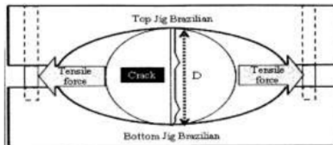
Gambar 4 Sampel batu uji kuat tarik Brazilian dan susunan jig (Rai dkk, 2014)
