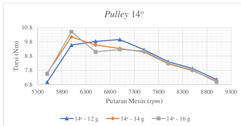
Gambar 3. Hasil Pengujian Sudut Pulley 14° dan Massa Rol 12 g, 14 g, & 16 g
