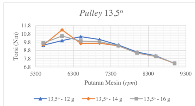
Gambar 2. Hasil Pengujian Sudut Pulley 13,5^\circ dan Massa Rol 12 g, 14 g, & 16 g
