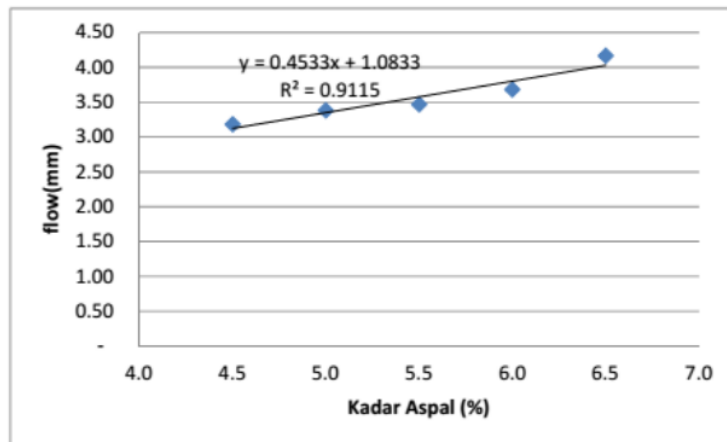
Gambar 8d. Grafik Hubungan Kadar Aspal dengan Flow
