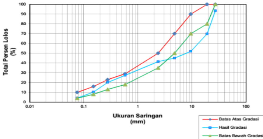
Gambar 4. Grafik gradasi agregat Kandang Mbelang
