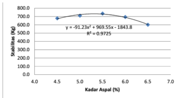
Gambar 8.c. Grafik Hubungan Kadar Aspal dengan Stabilitas
