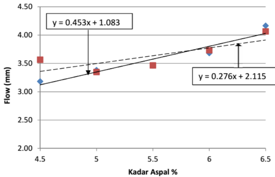
Gambar 9. Grafik Komparasi Nilai Flow
