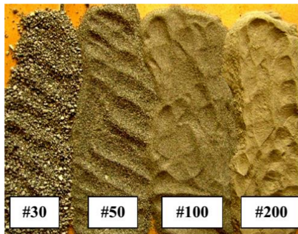
Gambar 6. Kenampakan visual agregat halus
