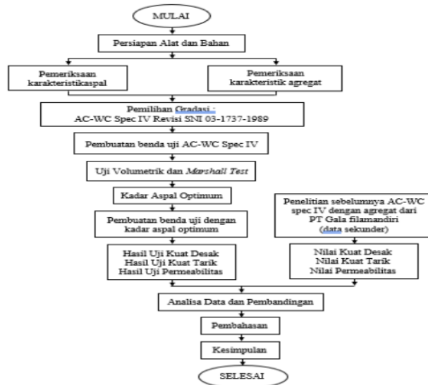
Gambar 1. Diagram alir tahapan penelitian
