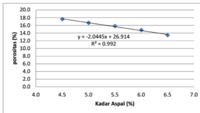
Gambar 8b. Grafik Hubungan Kadar Aspal dengan Porositas
