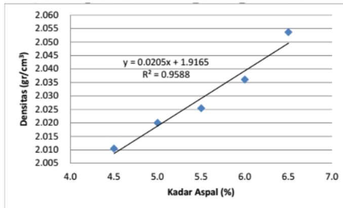
Gambar 8.a. Grafik Hubungan Kadar Aspal dengan Densitas
