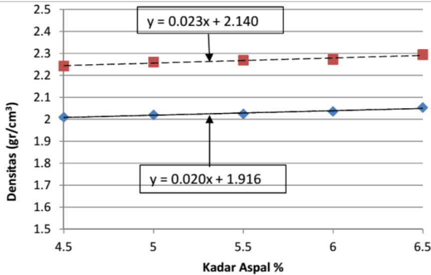
Gambar 10. Grafik Komparasi Nilai Densitas
