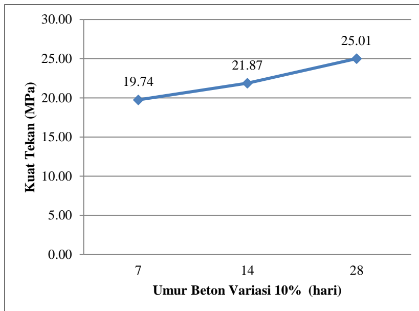
Gambar 6. Grafik pengujian kuat tekan variasi 10%
