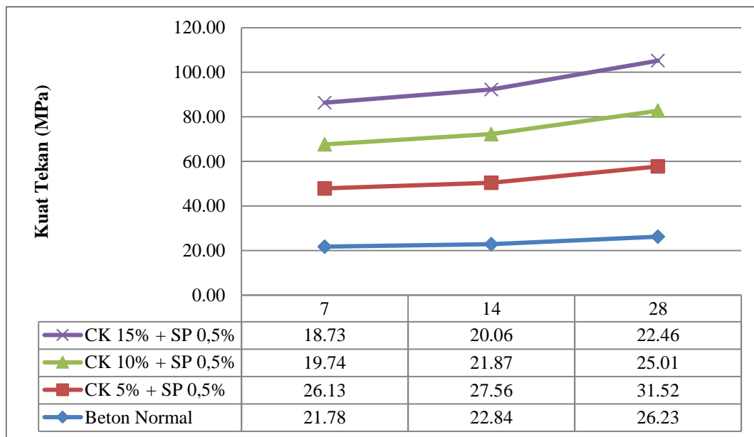
Gambar 8. Grafik gabungan kuat tekan variasi cangkang kerang
