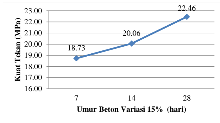
Gambar 7. Grafik pengujian kuat tekan variasi 15%
