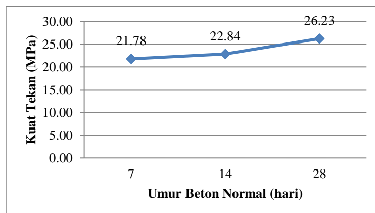
Gambar 4. Grafik pengujian kuat tekan beton normal
