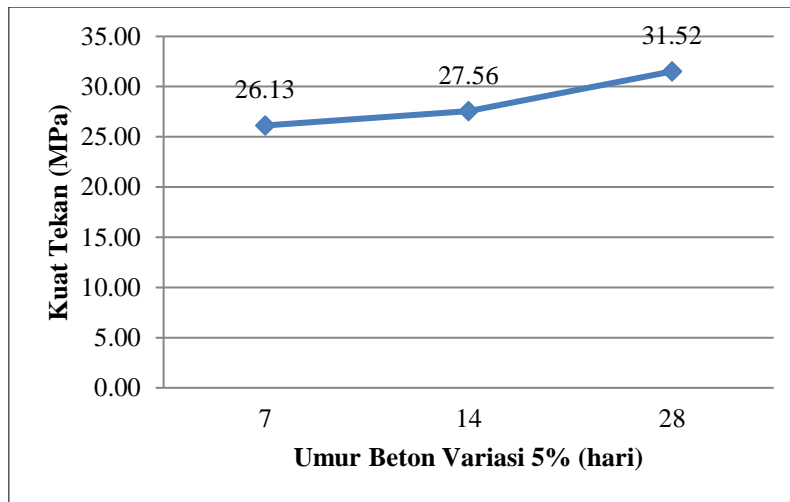
Gambar 5. Grafik pengujian kuat tekan variasi 5%
