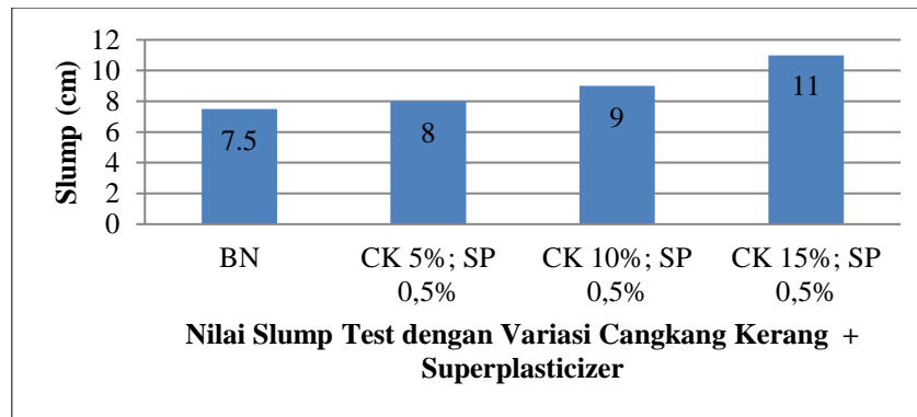
Gambar 3. Hubungan antara variasi campuran dengan nilai slump
