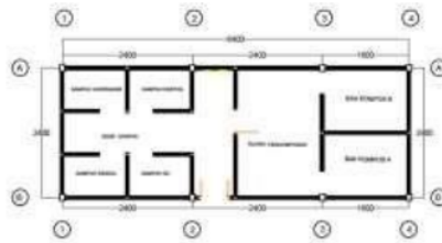
Gambar 16 Denah Bangunan Bank Sampah Sumber : Analisa Pribadi ( 2024 )
