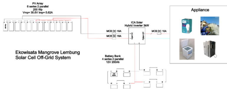
Gambar 3. Skema Sistem PLTS
