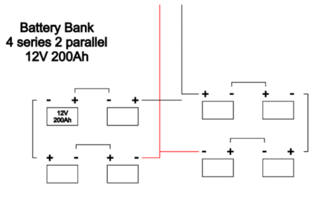
Gambar 2. Rangkaian Baterai
