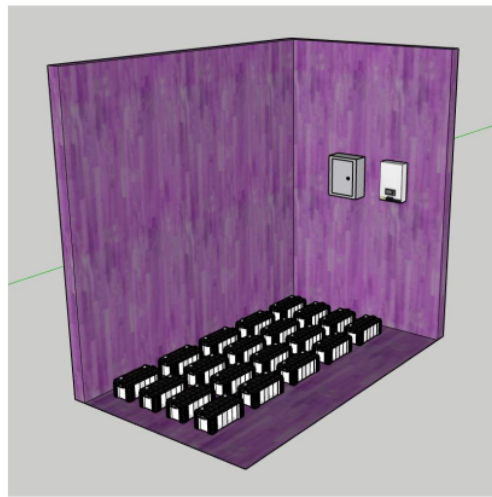
Gambar 6. Desain Ruang Penyimpanan Energi
