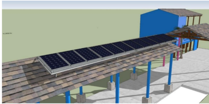
Gambar 5. Desain Atap PLTS Ekowisata Mangrove Lembung
