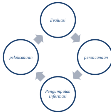
Gambar 1. Tahap Kegiatan
